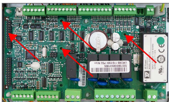
3. La carte d'extension doit être branchée à la prise CN9, et les fiches de la carte d'extension doivent être montées dans les trous prévus sur la carte CTS602.
