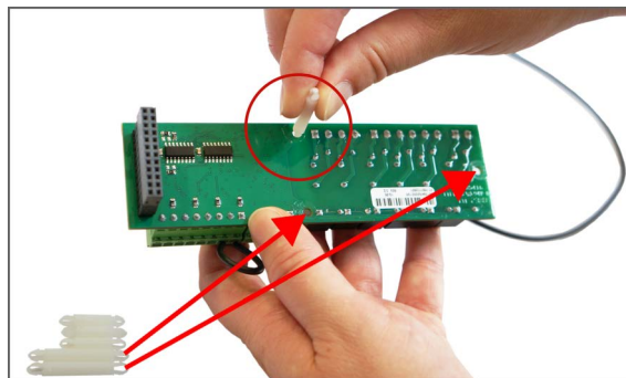
2. Installez les plus grandes fiches fournies (de la carte d'extension) dans les trois trous de la carte d'extension.
