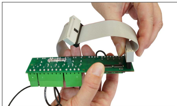
1. Débranchez le câble bus indiqué sur la carte d'extension.
