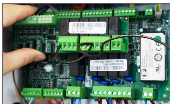
4. Installez la carte d'extension sur la carte électronique CTS602.
