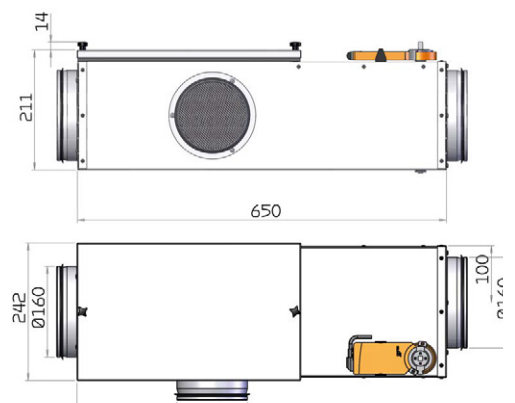
Schéma coté:
