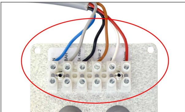
10b. Connectez le câblage comme indiqué ici et dans le schéma électrique suivant. La plaque peut être desserrée et accessible par le haut du Compact, ce qui peut faciliter l'installation.
