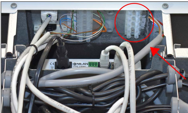
9. Faites passer le câblage devant le Gateway (Passerelle) avec les autres fils de la carte électronique et connectez-le au bornier de raccordement situé au-dessus du Compact.
