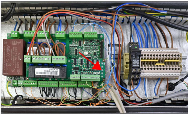
7. Installez la carte d'extension sur la carte électronique CTS602. Installez les autres câbles de la carte d'extension conformément au schéma électrique.
