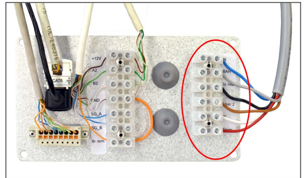
10a. Connectez le câblage comme indiqué ici et dans le schéma électrique suivant. La plaque peut être desserrée et accessible par le haut du Compact, ce qui peut faciliter l'installation.
