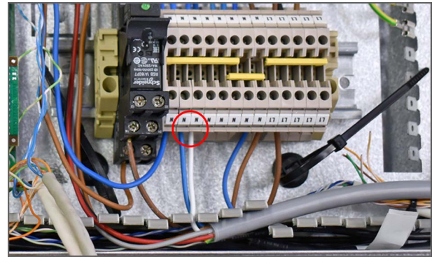
8. Connectez les fils blanc et bleu au fusible conformément au schéma électrique.
